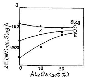
図2. 塩基度に対する \text{Al}_2\text{O}_3 添加の影響
