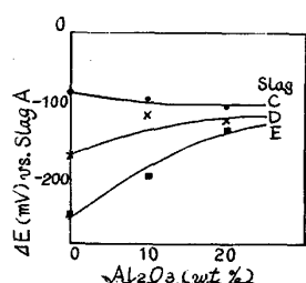
図2. 塩基度に対する \text{Al}_2\text{O}_3 添加の影響
