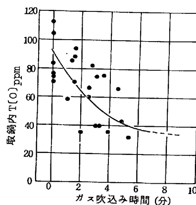
図1. ガス吹込み中の取鍋内酸素の変化
