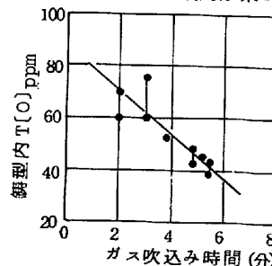
図2. ガス吹込み時間と鑄型内酸素との関係
