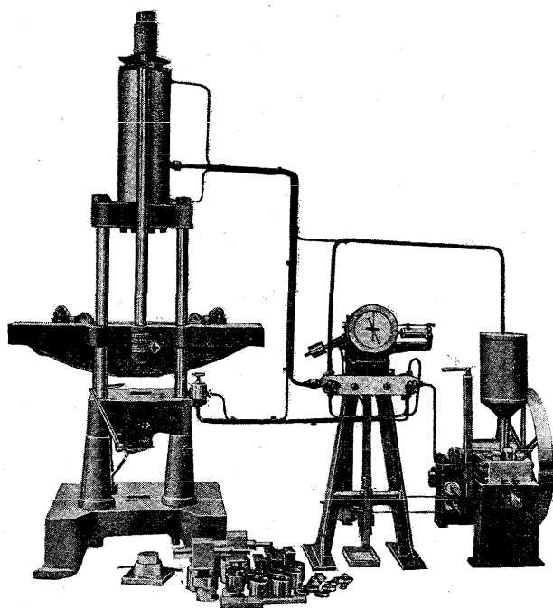
五拾五 東 京 衡 機 式 萬 能 強 弱 試 驗 機 材 料
