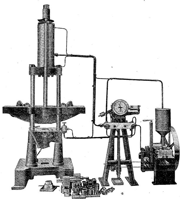
五拾噸 東 京 衡 機 強 弱 試 驗 機 能 萬 式 材 料 機 驗
