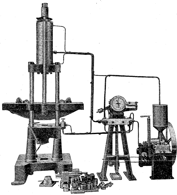
五拾貳式萬能試驗機 東京衡機 強弱試驗材料
