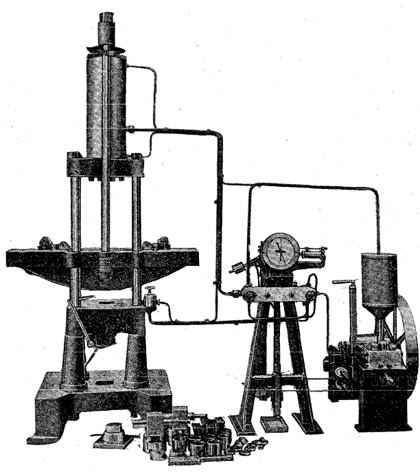
五拾貳 東 京 衡 機 槓 桿 式 萬 能 材 料 強 弱 試 驗 機
